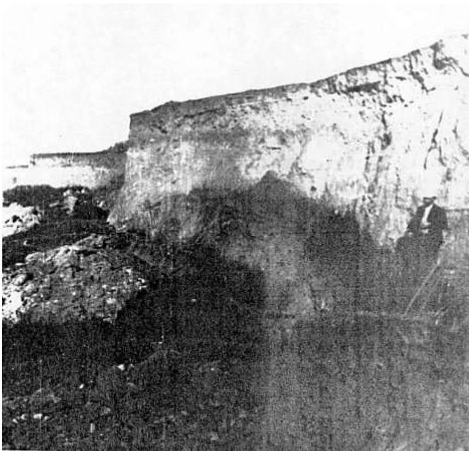
Рис. 2.1.2. Грандиозный срыв горных пород в результате землетрясения. Фото Лейбница (Мушкетов, 1887)
