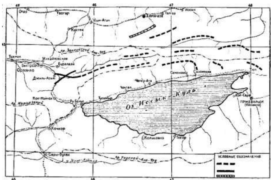
Рис. 2.1.3. Распределение линий разломов во время Верненского 1887 г. (3), Кеминского 1911 г. (1) и Кемино-Чуйского 1938 г. (2) землетрясений (Богданович и др., 1914)
