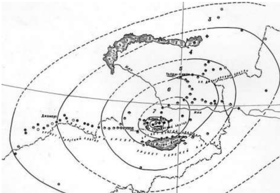
Рис. 2.1.4. Распределение силы сотрясений Верненского землетрясения 1887 г.
