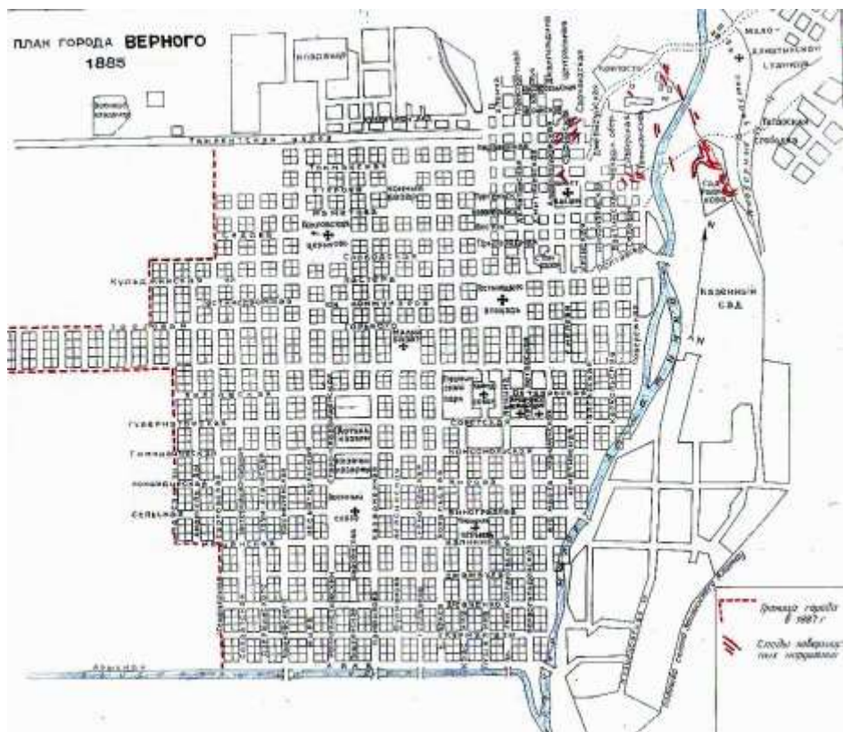
Рис. 2.1.18. Распределение силы сотрясений Верненского землетрясения по территории г. Верного
